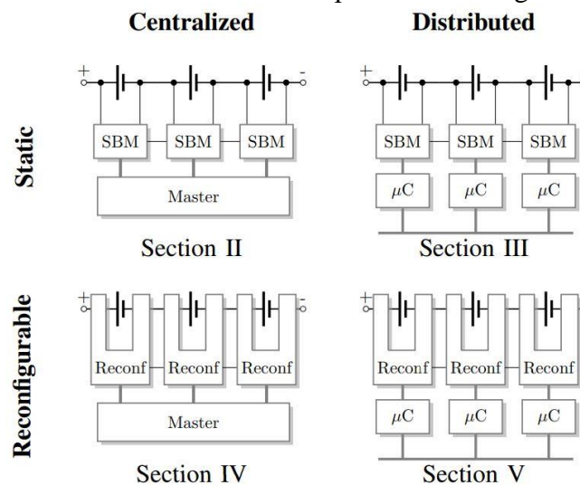
Figura 1 Clasificarea arhitecturilor de management a bateriilor [15]
