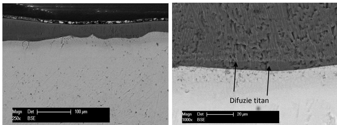
Fig. 13 Micrografii MEB ale stratului \text{Al}_2\text{O}_3\text{-TiO}_2 depus prin metoda HVOF si retopit cu fascicul de electroni
