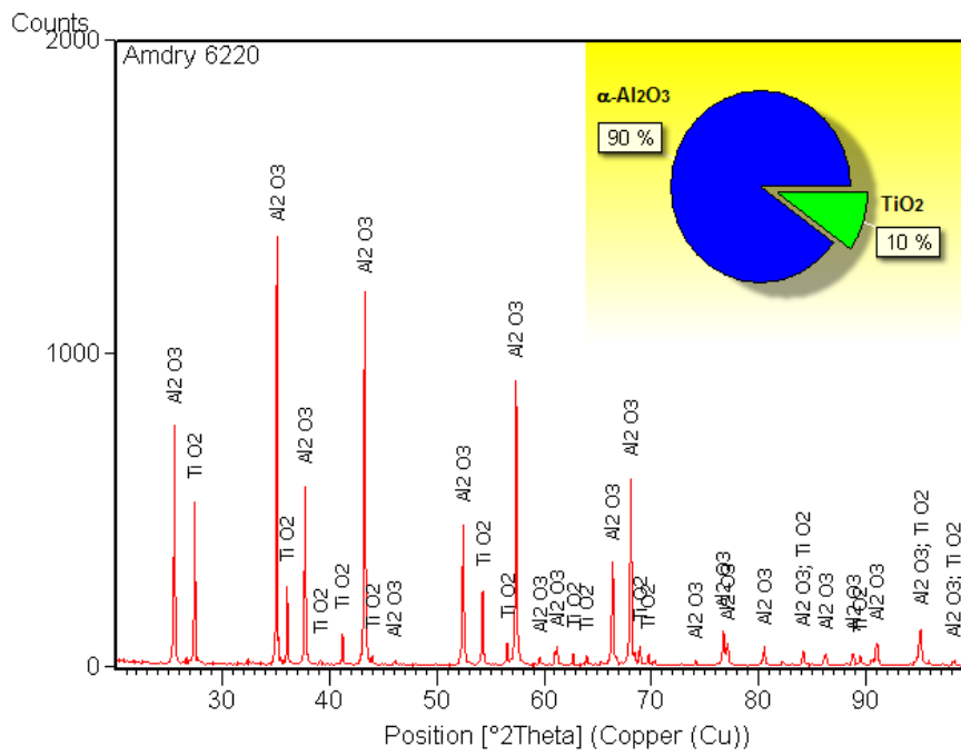
Fig. 15 Spectru RX al pulberii \text{Al}_2\text{O}_3\text{-TiO}_2
