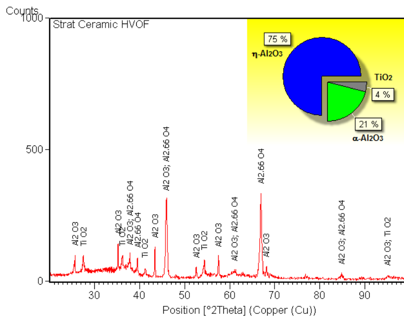
Fig. 16 Spectru RX al stratului \text{Al}_2\text{O}_3\text{-TiO}_2 pulverizat HVOF
