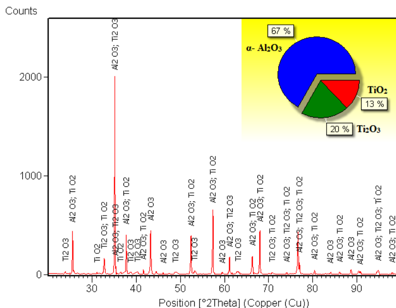
Fig. 19 Spectru RX al stratului \text{Al}_2\text{O}_3 - \text{TiO}_2 pulverizat APS si retopit cu fascicul de electroni
